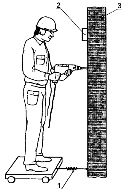
1 — горизонтальный динамометр или силовая платформа; 2 — устройство для считывания усилия подачи; 3 — вертикальная бетонная стена
